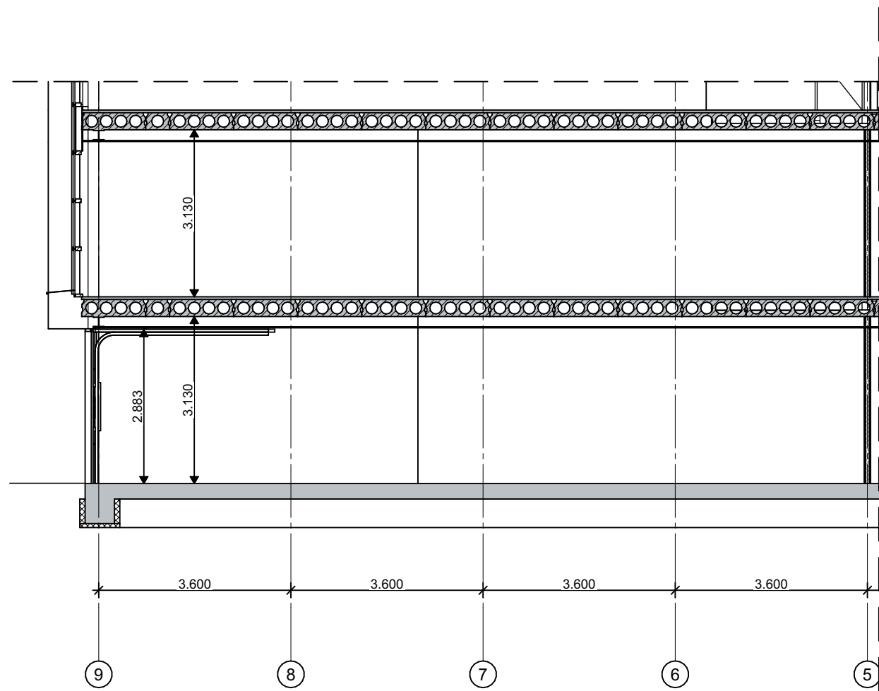
Doorsnede BB nieuw schaal 1:100
