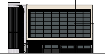
Doorsnede EE nieuw schaal 1:100
