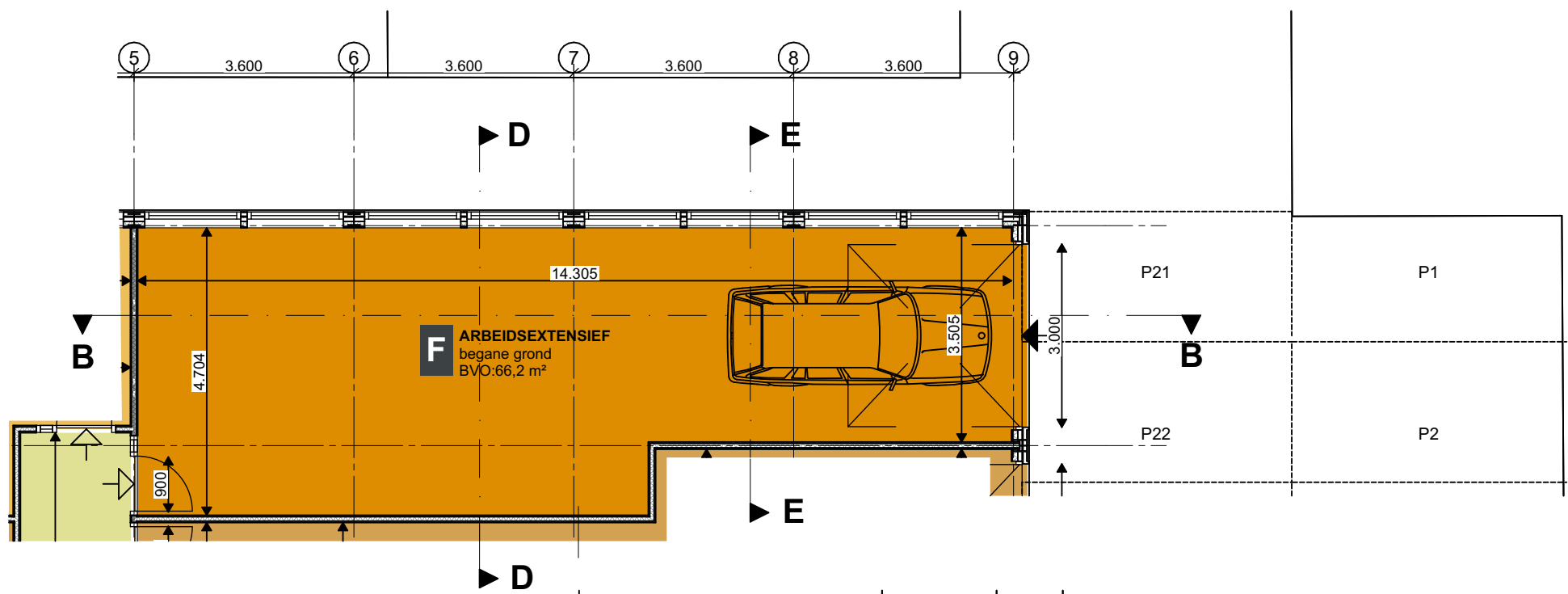
Begane grond nieuw schaal 1:100
