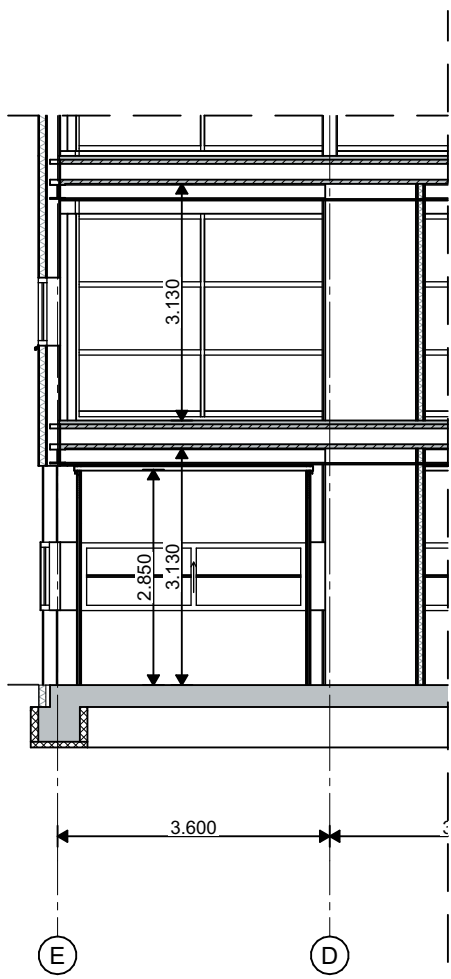
Doorsnede DD nieuw schaal 1:100
