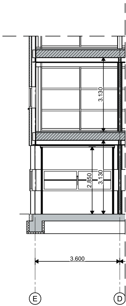
Doorsnede EE nieuw schaal 1:100
