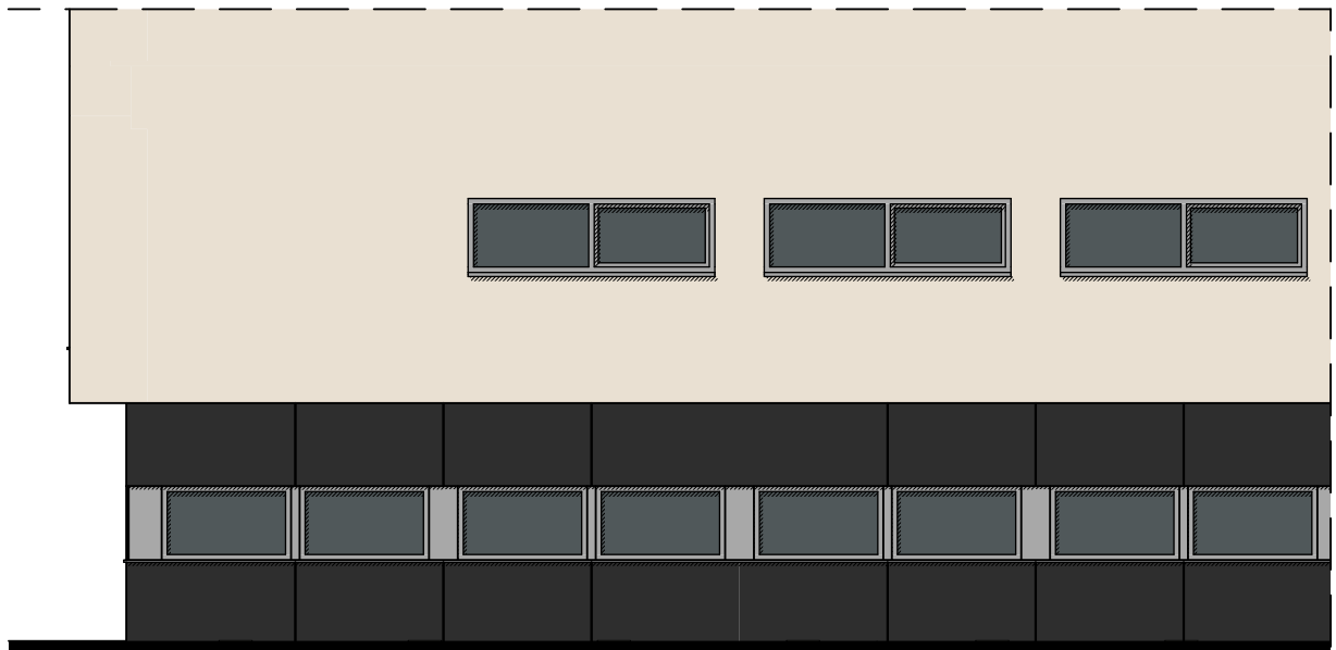
Oostgevel nieuw schaal 1:100
