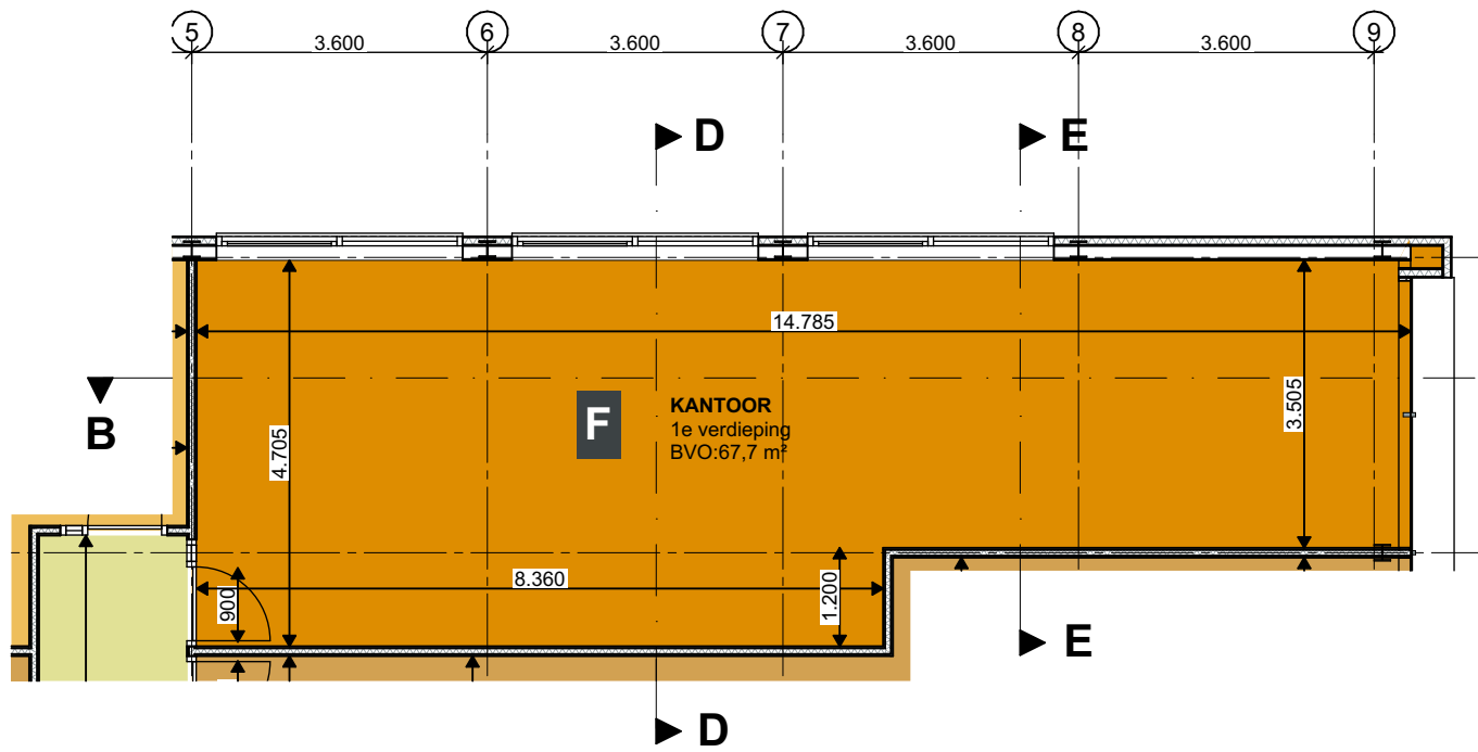
1e verdieping schaal 1:100
